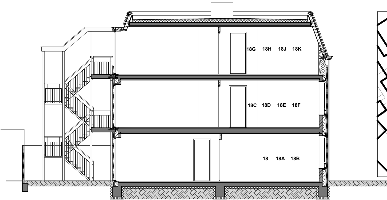
doorsnede
