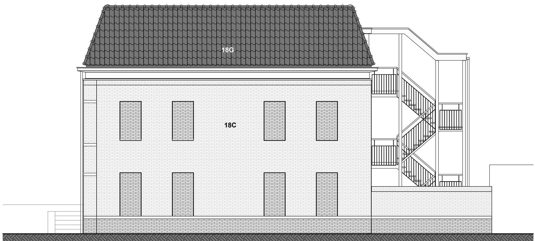
zij aanzicht
